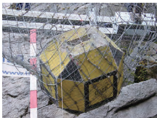
補修したネットで再度捕捉
