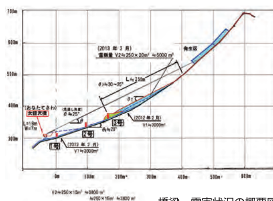
橋梁・雪害状況の概要図
