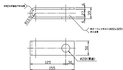
アンカーバンド詳細図 (SS400相当)
