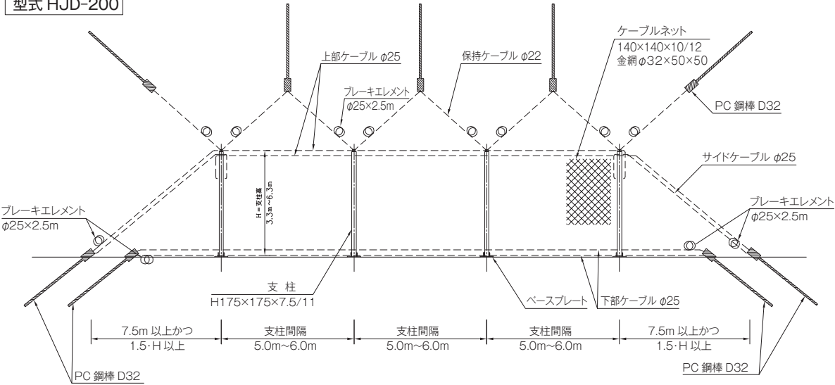
(例) 型式 HJD-200
