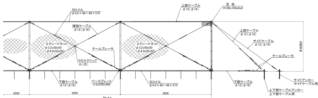
正面図
