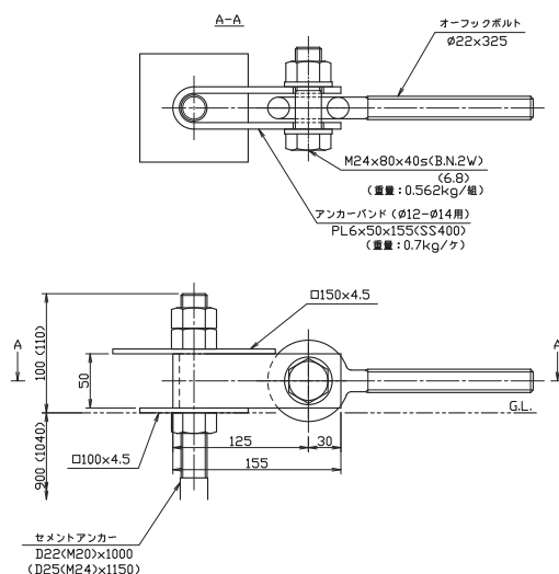
設置図
