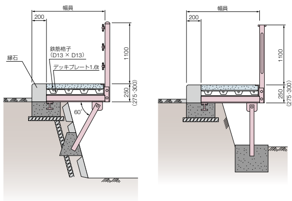
Aタイプ(支柱傾斜)
