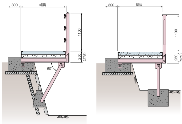
Aタイプ(支柱傾斜)
