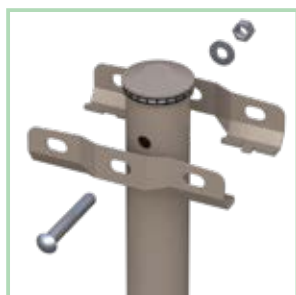
標準・端部ブラケットの取付け
