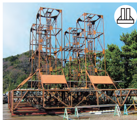
E600L-2 石詰付き (H10m×WL12m)
