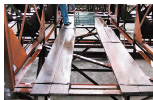
足場板敷設
