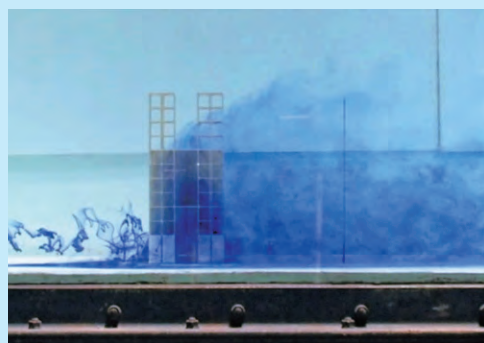
湧昇イメージ(水槽実験)
