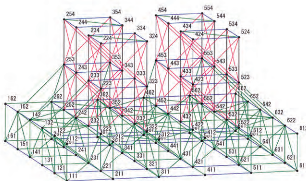
解析モデル例
