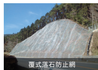
ケーブルネット
