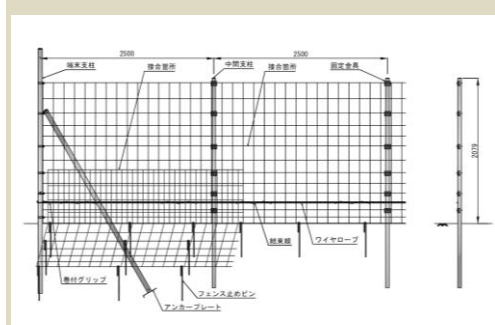
シカ・イノシシ防護柵
