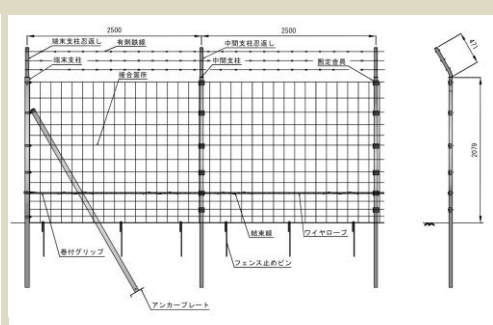
シカ防護柵 忍び返し付
